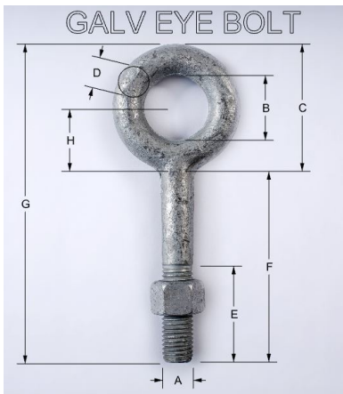
Galv eye bolt
